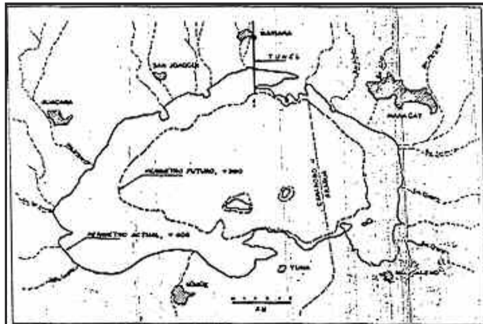
FIGURA 3. Bajando el nivel del lago de Valencia de la cota actual (aprox. 405 m) a la cota 380 m, la superficie lacustre pasaría de los actuales 340km 2 (línea continua) a 175 km 2 (línea punteada) y se obtendrían 16.500 hectáreas de nuevas tierras.
